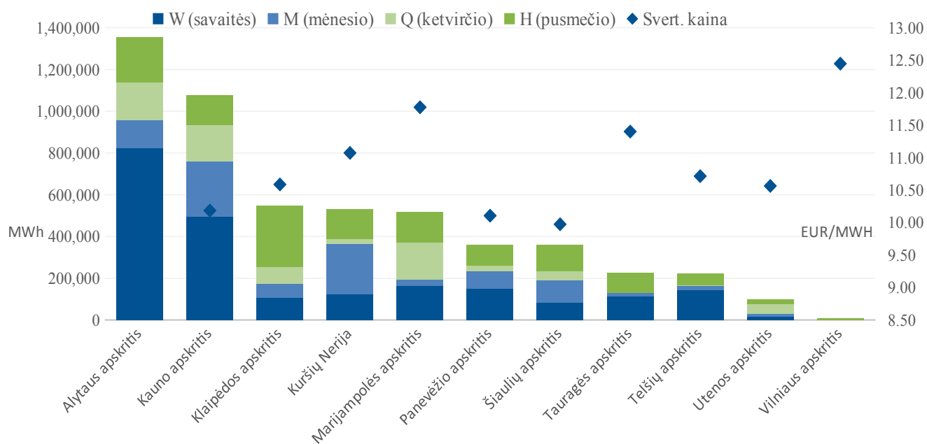
Pav. 4. Per ataskaitinį laikotarpį pagal biokuro biržoje sudarytus sandorius faktiškai pristatytų medienos skiedros produktų kiekiai (MWh) apskrityse pagal sandorių trukmę ir vidutinę medienos skiedros produktų tiekimo kainą (Eur/MWh)
