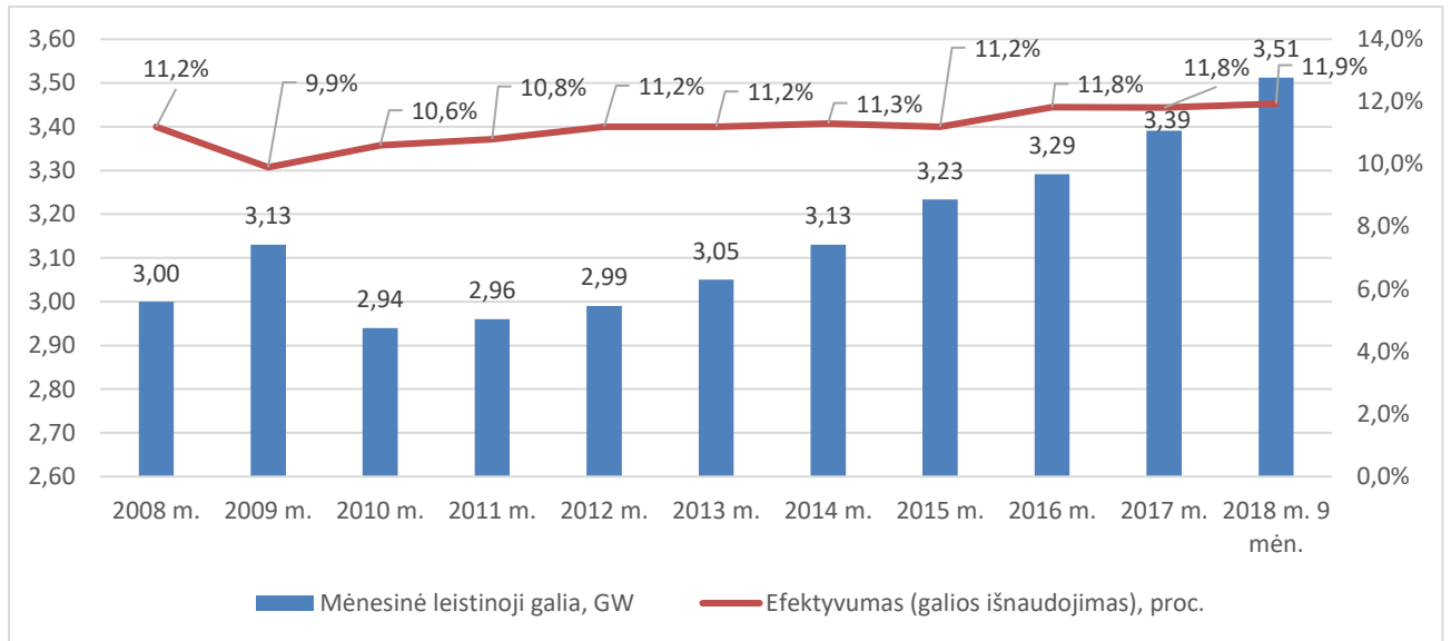
2 pav. Bendrovės komercinių vartotojų leistosios naudoti galios ir jos išnaudojimo dinamika ŽĮ tinkluose
