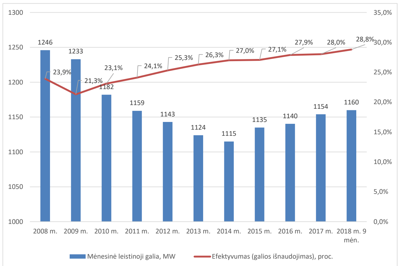
1 pav. Bendrovės komercinių vartotojų leistosios naudoti galios ir jos išnaudojimo dinamika VĮ tinkluose
