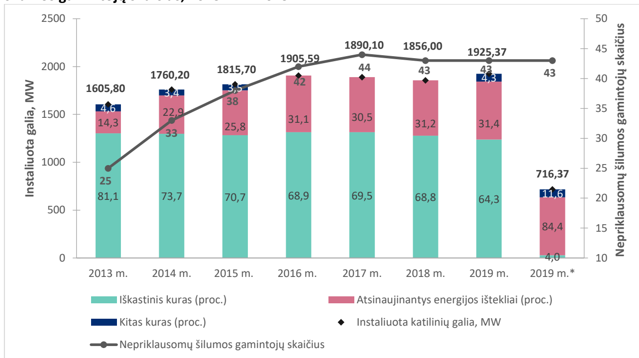
1 pav. Instaliuota katilinių galia pagal šilumos gamybai naudojamą kurą (MW) ir nepriklausomų šilumos gamintojų skaičius, 2013 m. – 2019 m.
