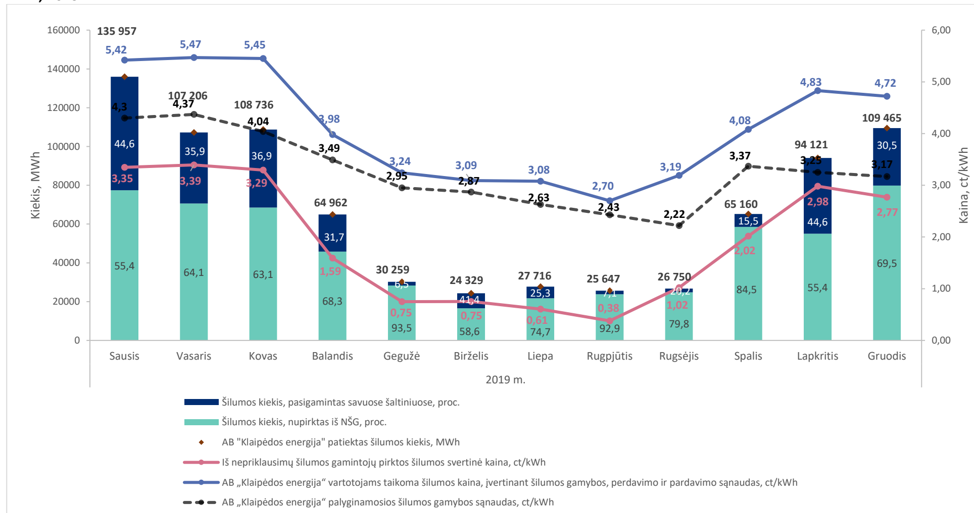
13 pav. Nepriklausomų šilumos gamintojų parduotos šilumos dalis AB „Klaipėdos energija“ patiektoje į tinklą šilumos struktūroje, proc., parduotos šilumos kaina ir AB „Klaipėdos energija“ vartotojams parduodamos šilumos kaina, ir palyginamosios šilumos gamybos sąnaudos euro ct/kWh be PVM, 2019 m.
