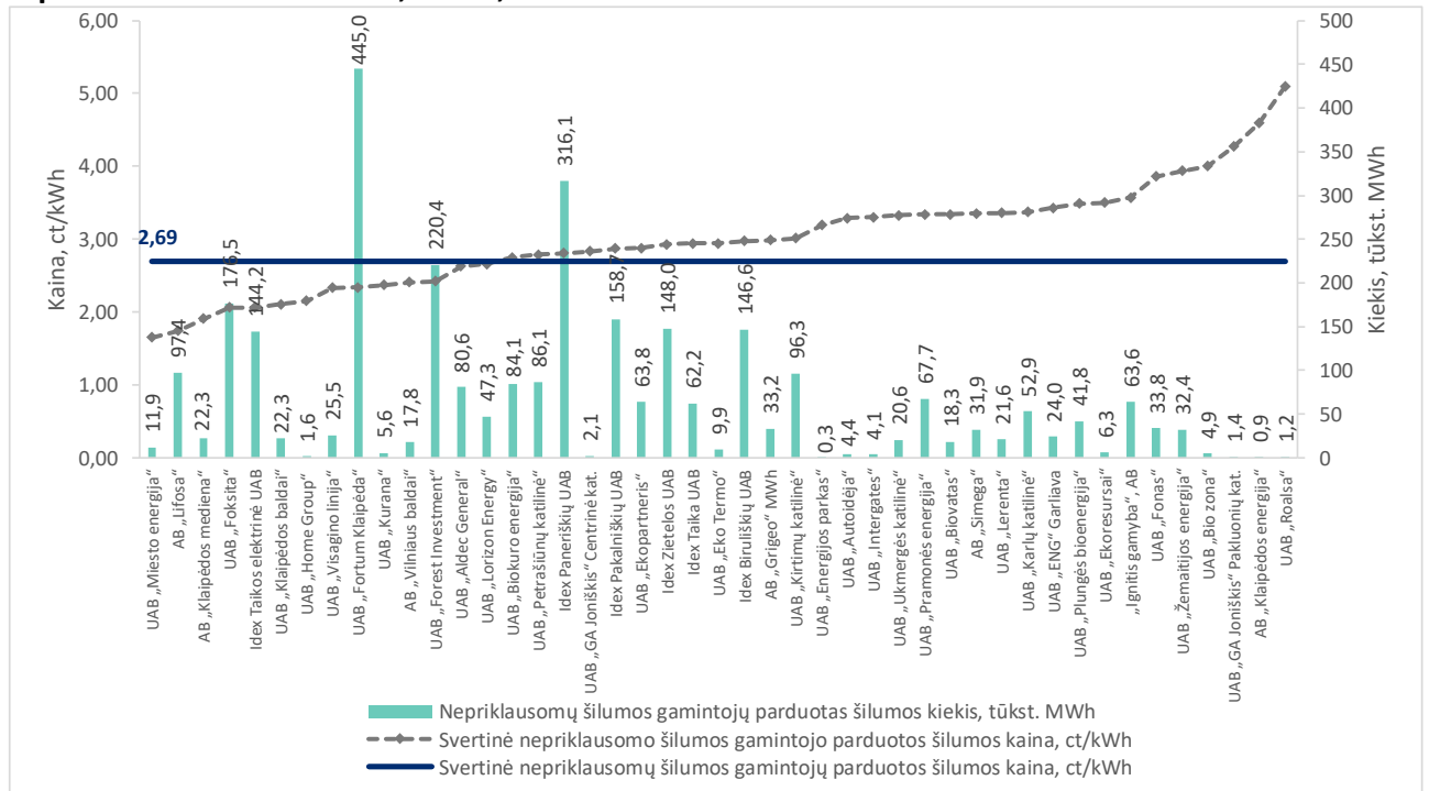
7 pav. Svertinė nepriklausomų šilumos gamintojų parduotos šilumos kaina, euro ct/kWh be PVM ir parduotos šilumos kiekis, MWh, 2019 m.
