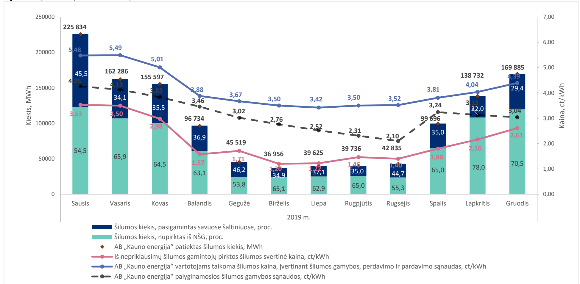
12 pav. Nepriklausomų šilumos gamintojų parduotos šilumos dalis AB „Kauno energija“ Kauno miesto sistemoje patiektos į tinklą šilumos struktūroje, proc., parduotos šilumos kaina ir AB „Kauno energija“ vartotojams parduodamos šilumos kaina ir palyginamosios šilumos gamybos sąnaudos, euro ct/kWh be PVM, 2019 m.
