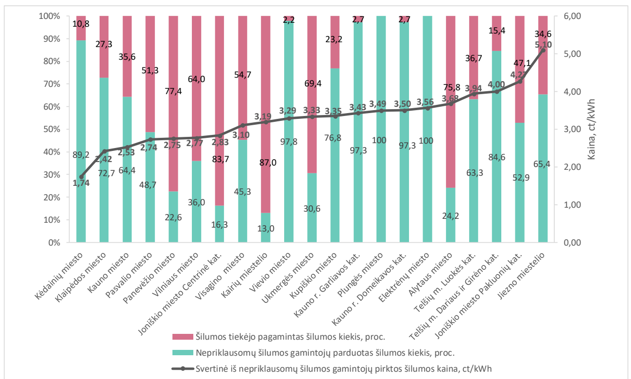
8 pav. Nepriklausomų šilumos gamintojų parduotos šilumos dalis CŠT sistemoje ir svertinė kaina 2019 m.
