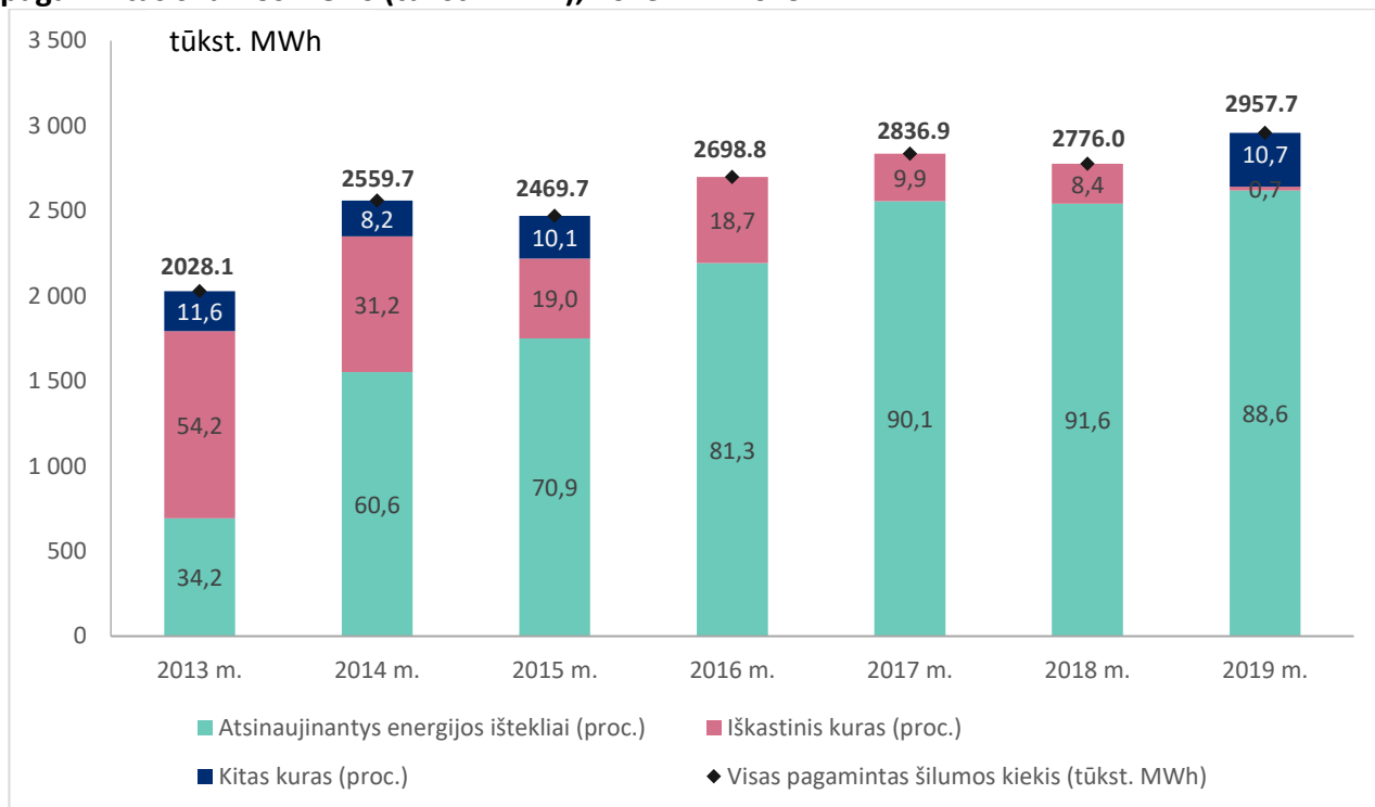
3 pav. Nepriklausomų šilumos gamintojų pagamintos šilumos kiekis pagal kuro rūšis (proc.) ir visas pagamintas šilumos kiekis (tūkst. MWh), 2013 m.– 2019 m.
