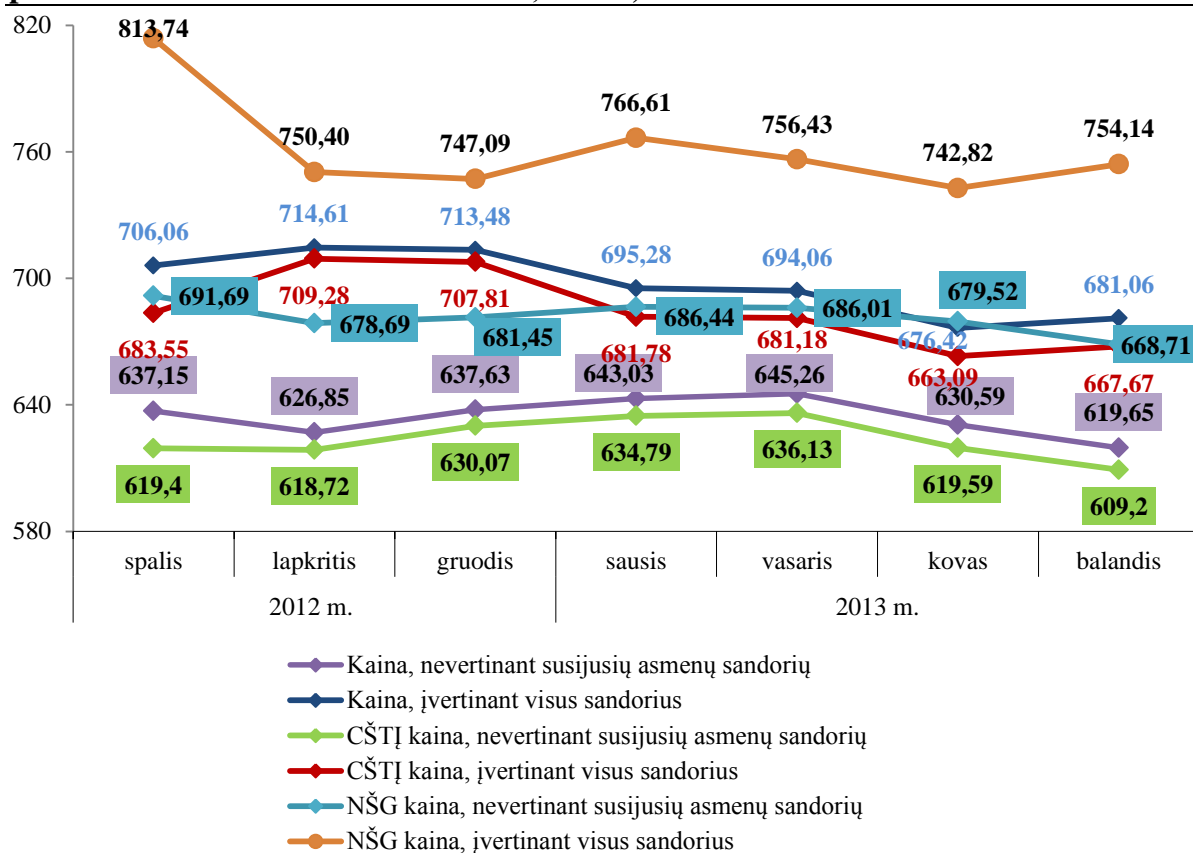
5 pav. Nepriklausomų šilumos gamintojų ir Komisijos licencijuojamų šilumos tiekėjų pirko biokuro vidutinė svartinė kaina, Lt/tne, 2012–2013 metai
