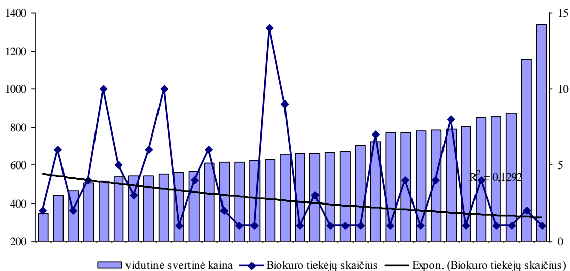
12 pav. Komisijos licencijuojamų šilumos tiekėjų pirktų biokuro kainos Lt/tne ir biokuro tiekėjų skaičiaus priklausomybė, 2012–2013 metų šildymo sezonas.
