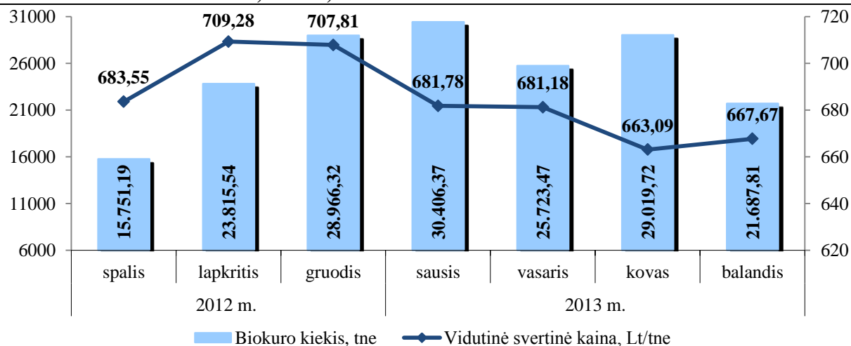
9 pav. Komisijos licencijuojamų šilumos tiekėjų pirko biokuro kiekiai*, tne ir vidutinės svertinės kainos dinamika**, Lt/tne, 2012–2013 metai
