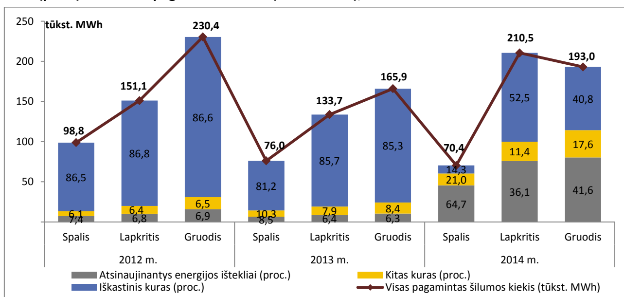
2 pav. Reguliuojamų nepriklausomų šilumos gamintojų pagamintos šilumos kiekis pagal kuro rūšis (proc.) ir bendras pagamintas kiekis (tūkst. MWh), 2012 m. IV ketv. – 2014 m. IV ketv.
