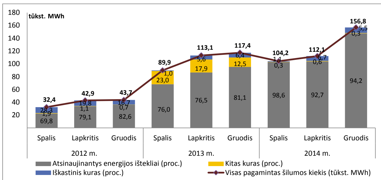
3 pav. Nereguliuojamų nepriklausomų šilumos gamintojų pagamintos šilumos kiekis pagal kuro rūšis (proc.) ir bendras pagamintas kiekis (tūkst. MWh), 2012 m. IV ketv. – 2014 m. IV ketv.
