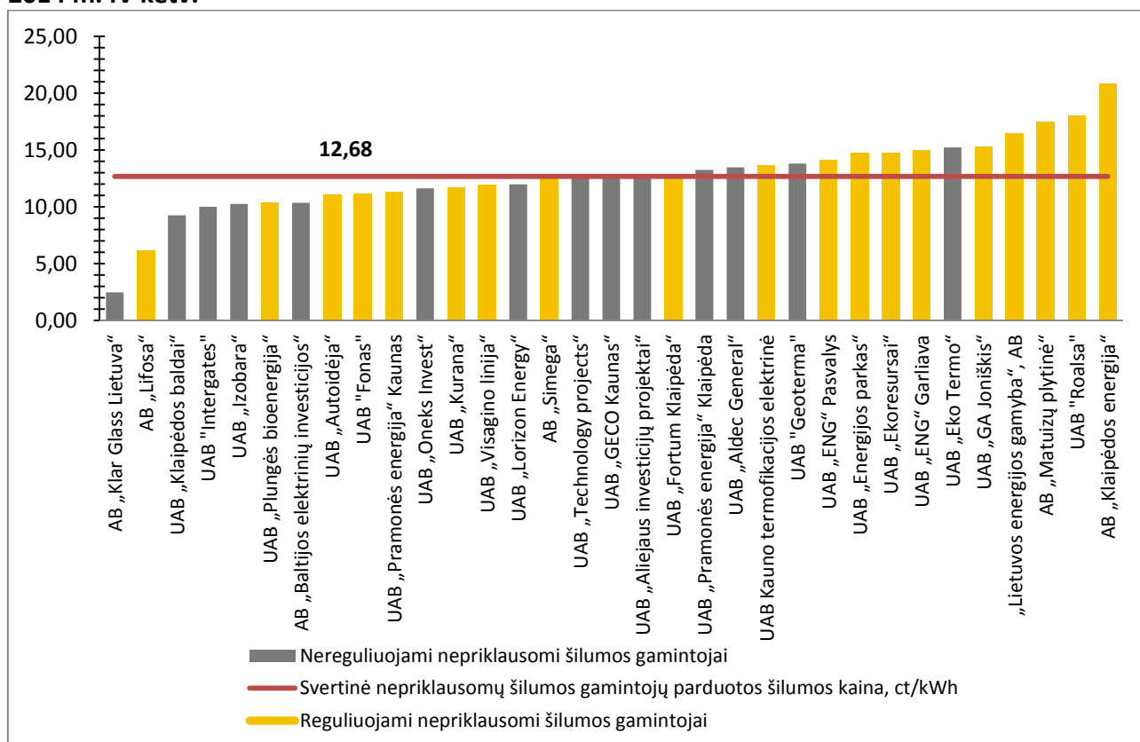
18 pav. Svertinė nepriklausomų šilumos gamintojų parduotos šilumos kaina, ct/kWh be PVM, 2014 m. IV ketv.
