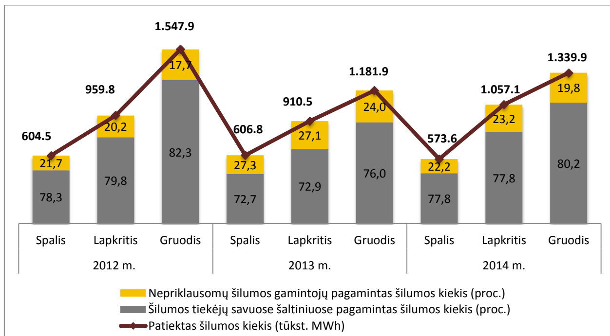
6 pav. Nepriklausomų šilumos gamintojų ir Komisijos licencijuojamų šilumos tiekėjų vartotojams patiekto šilumos kiekio struktūra, 2012 m. IV ketv. – 2014 m. IV ketv.
