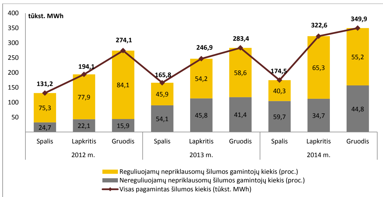
1 pav. Reguluojamų ir nereguluojamų nepriklausomų šilumos gamintojų pagamintos šilumos dalis (proc.) ir bendras pagamintas kiekis (tūkst. MWh), 2012 m. IV ketv. – 2014 m. IV ketv.
