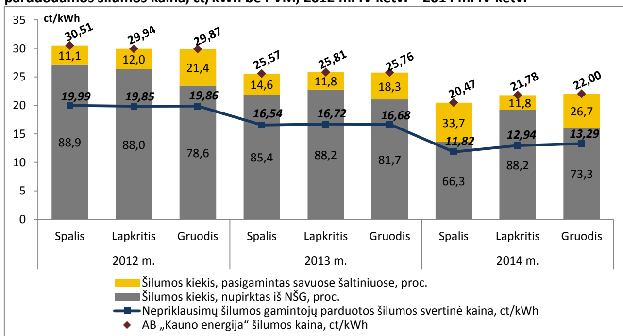
13 pav. Nepriklausomų šilumos gamintojų parduotos šilumos dalis AB „Kauno energija“ patiektos į tinklą šilumos struktūroje, proc., parduotos šilumos kaina ir AB „Kauno energija“ parduodamos šilumos kaina, ct/kWh be PVM, 2012 m. IV ketv. – 2014 m. IV ketv.
