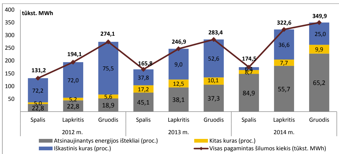
5 pav. Nepriklausomų šilumos gamintojų pagamintos šilumos kiekis pagal kuro rūšis (proc.) ir visas pagamintas šilumos kiekis (tūkst. MWh), 2012 m. IV ketv. – 2014 m. IV ketv.
