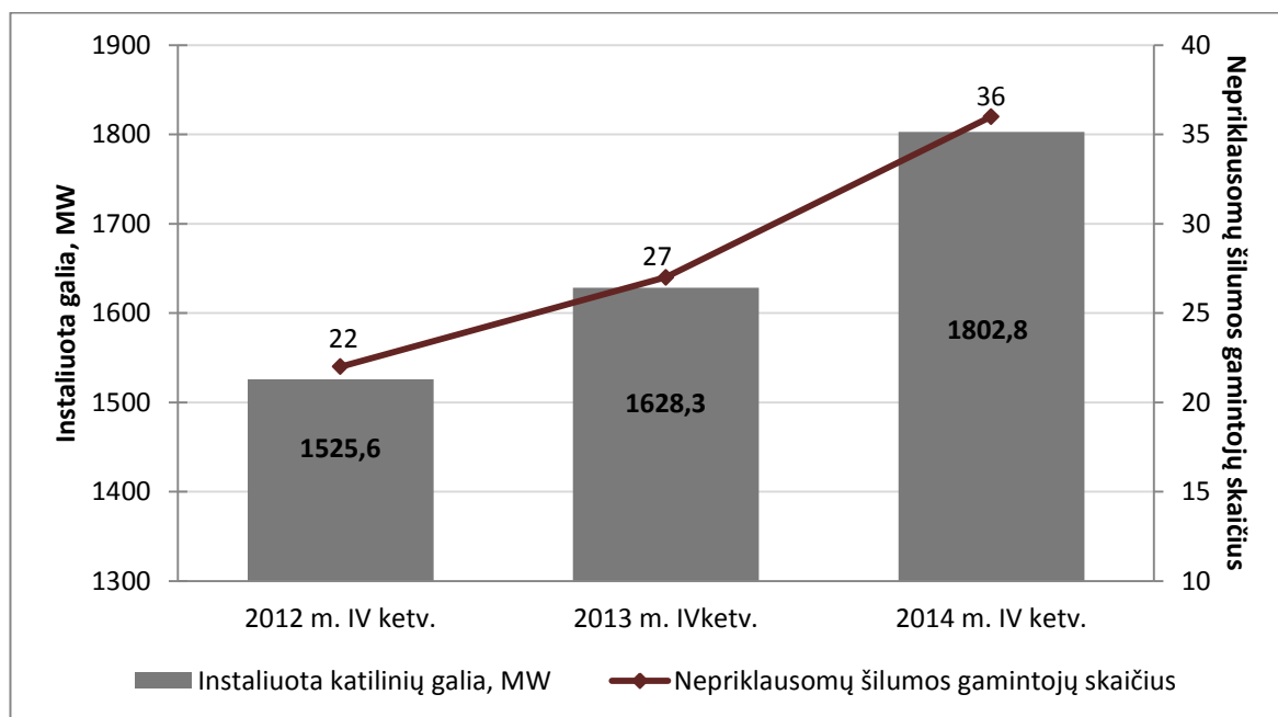
7 pav. Instaliuota katilinių galia (MW) ir nepriklausomų šilumos gamintojų skaičius, 2012 m. IV ketv. – 2014 m. IV ketv.
