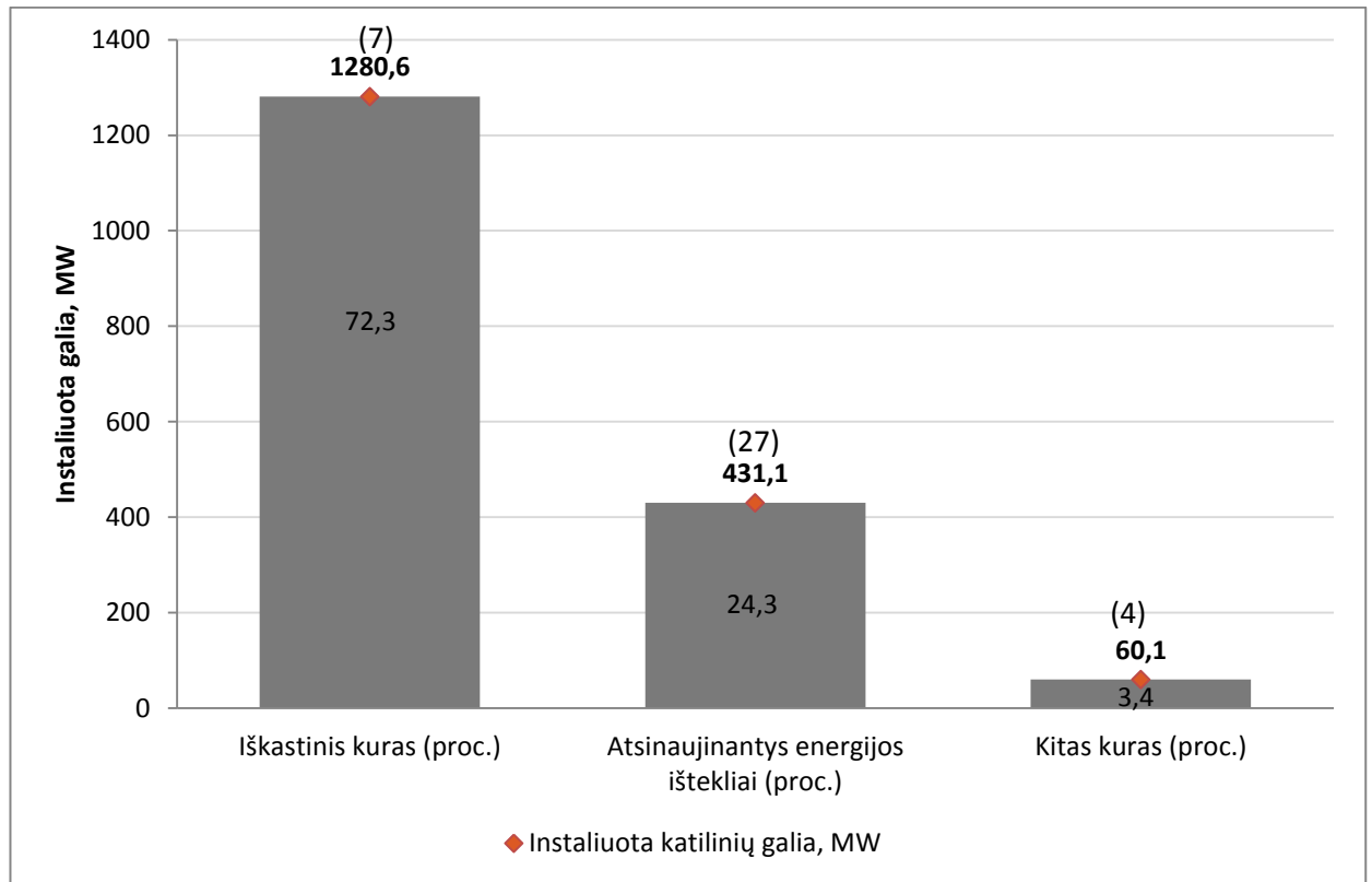
8 pav. Instaliuota katilinių galia pagal šilumos gamybai naudojamą kurą (MW) 2014 m. IV ketv.
